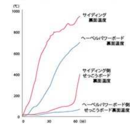
【外壁材裏面と内装せつこうボード裏面の温度変化】
